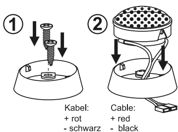
Abbildung 3 Aufbau Hochtöner Figure 3 Surface mount of Tweeter
